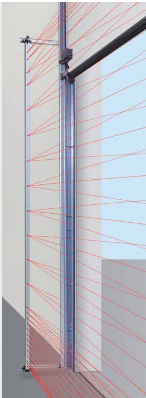
Montáž na zárubni vrat
