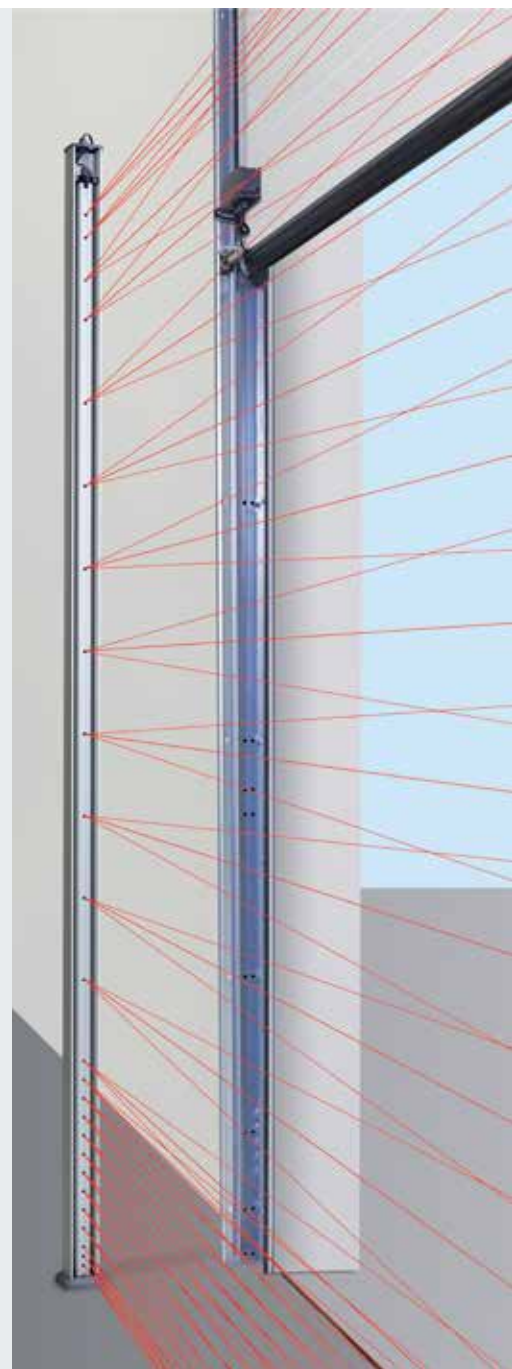
Montáž se sadou sloupků STL
